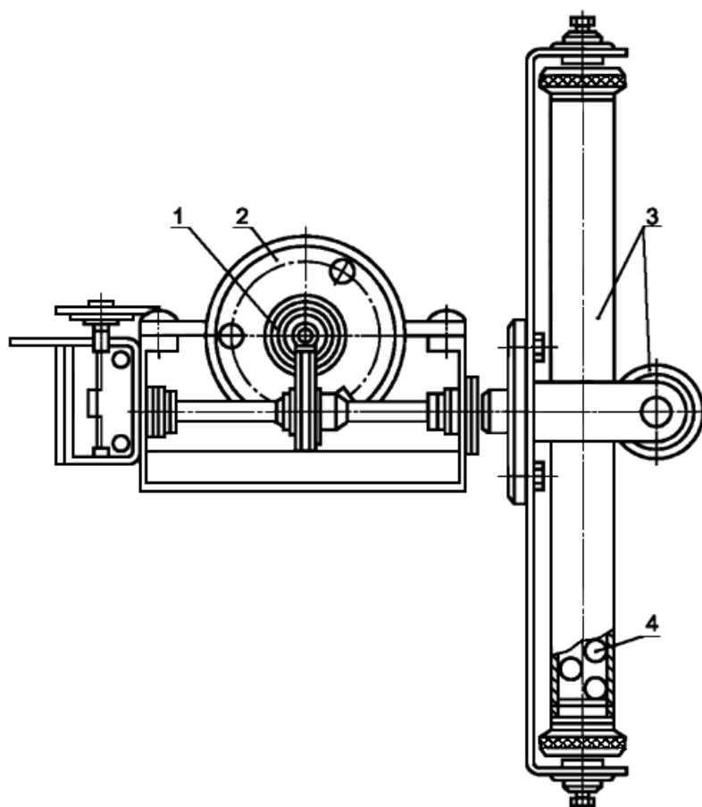
1 - редуктор; 2 - мотор; 3 - цилиндр; 4 - стальной шар
